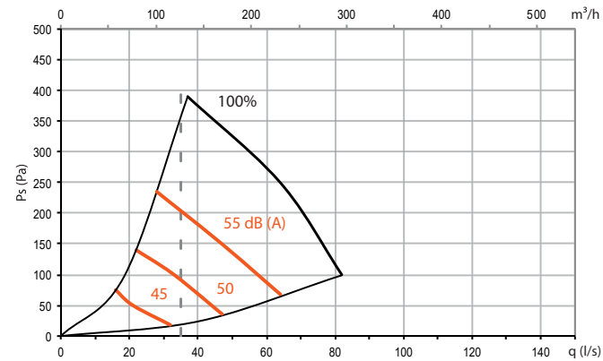
Ljudeffektnivå till kanal för köksförläng
