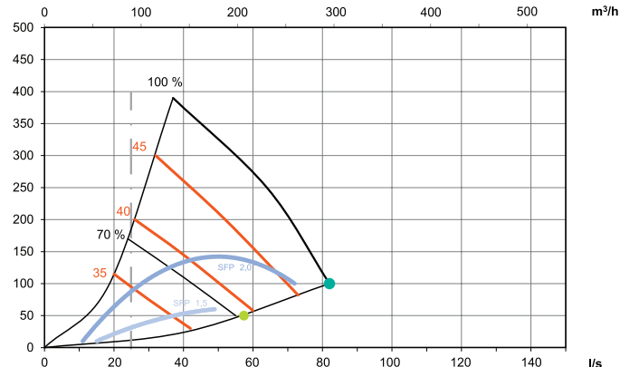
Luftflöde och ljudeffektnivå till omgivningen
