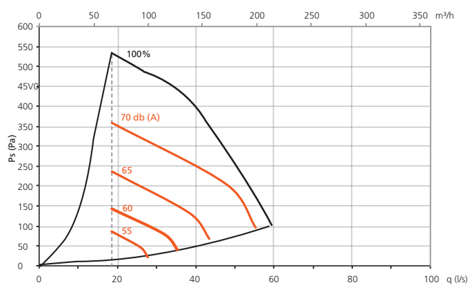
Ljudeffektnivå till avluftskanal
