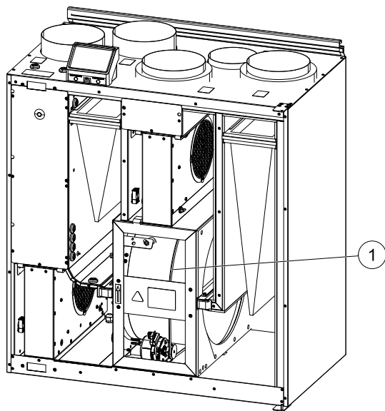
Fig. 6 Rotordrivrem
