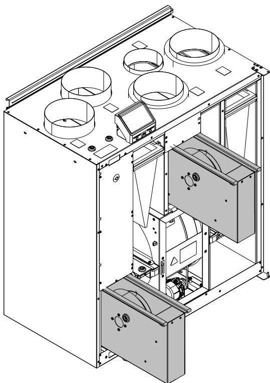
Fig. 5 Från- och tilluftsfläktar
