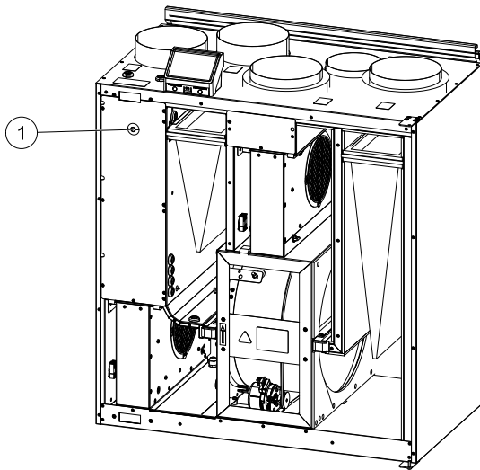
Fig. 7 Återställningsknapp för överhettningsskydd
