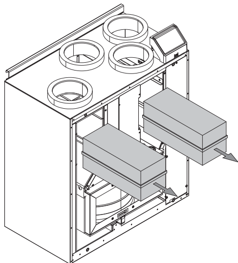
Fig. 4 Värmeväxlarfilter
