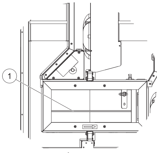
Fig. 7 Rotordrivrem
