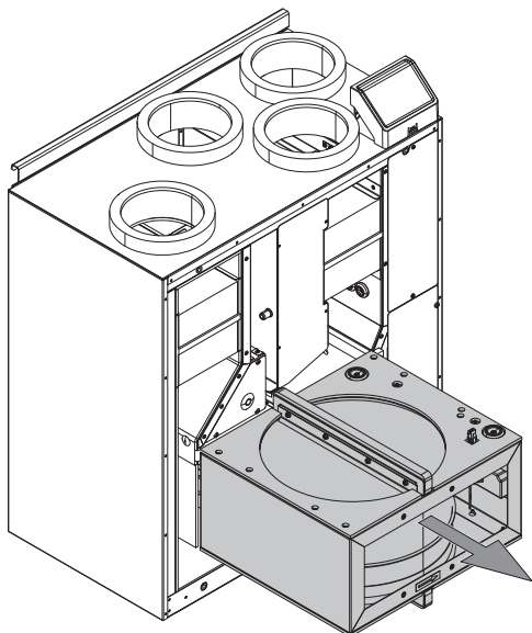
Fig. 5 Värmeväxlare
