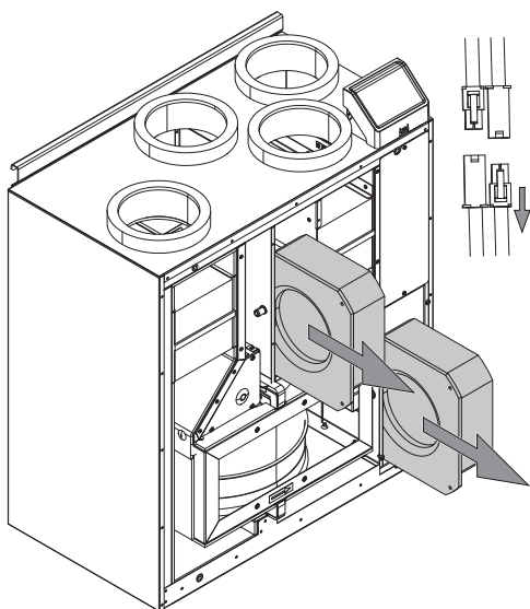
Fig. 6 Från- och tilluftsfläktar
