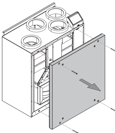
Fig. 3 Demontering/montering av invändig front
