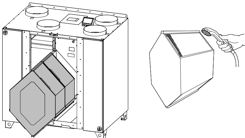
Fig. 7 Borttagning och rengöring av värmeväxlaren
