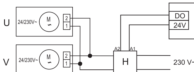
Fig. 16 Spjällanslutning
