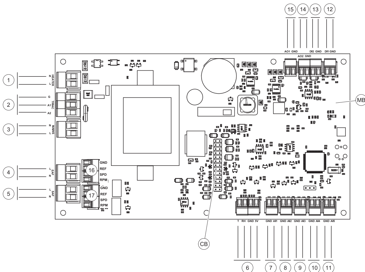
Fig. 4 Huvudkretskortet anslutningar
