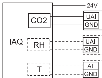
Fig. 11 IAQ-anslutningar
