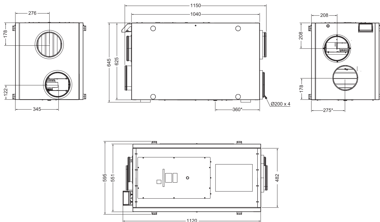
Fig. 2 Dimensioner för VSR 500
