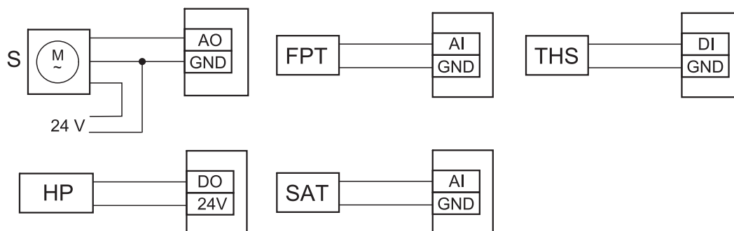
Fig. 15 Växlande uppvärmnings-/kylningsanslutningar
