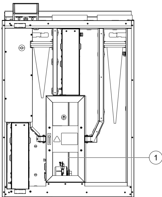
Fig. 6 Rotordrivrem
