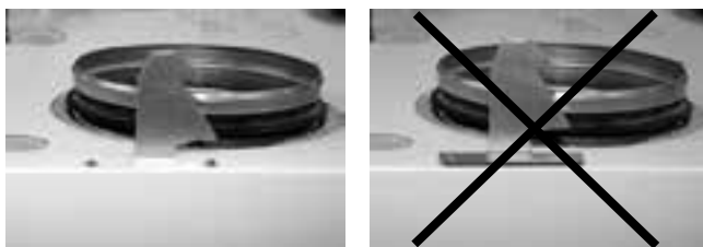
Krokarnas spetsar pekar mot aggregatets bakre del och de träns in i aggregatets urtag före nitningen.
