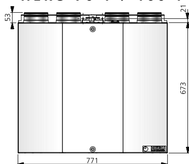
HERU®70 T / 100 T EC
